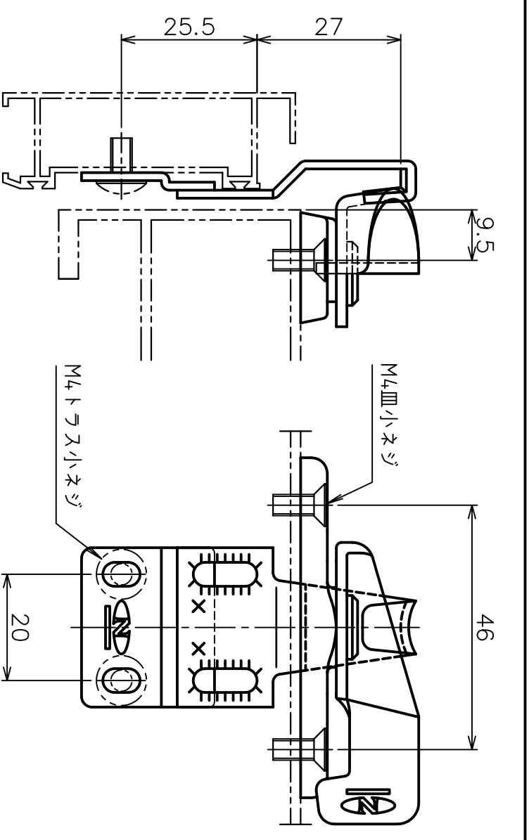
ステンレスクリセット / クリセット受け SUS-CL-100-01 (セット品番)
