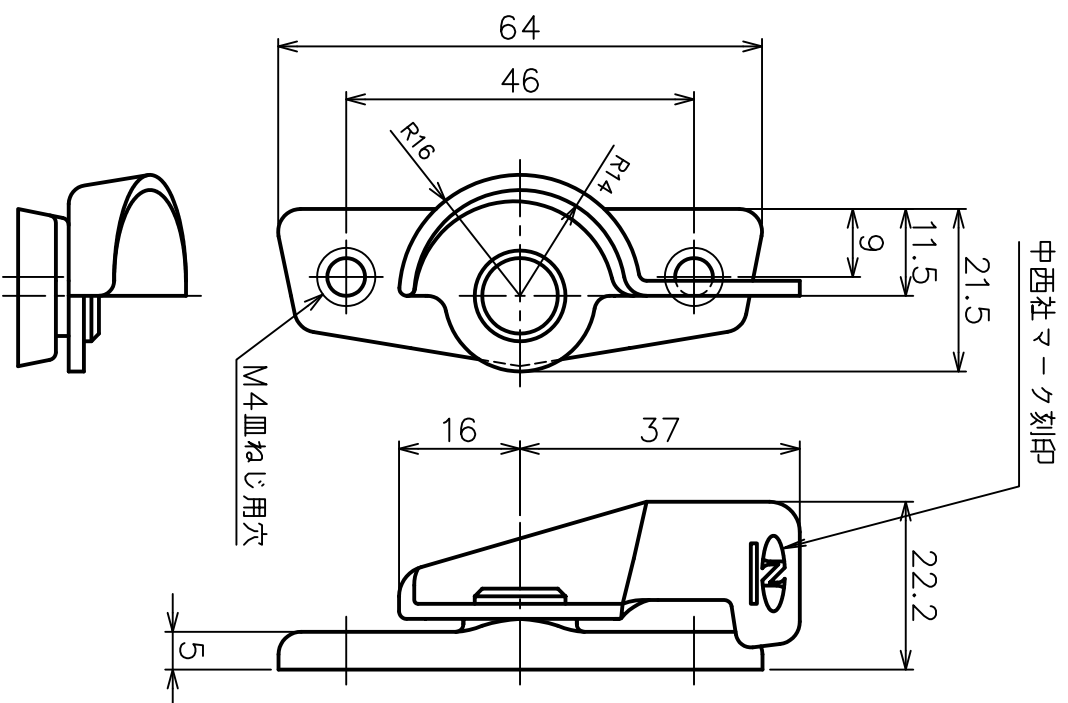
ステンレスクリセット (左勝手) SUS-CL-100
