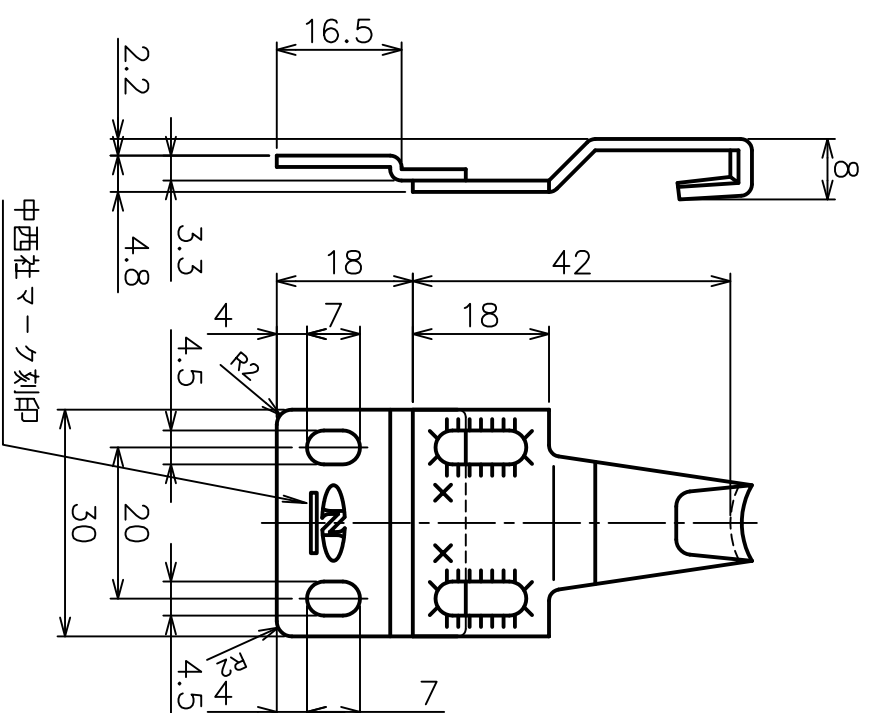
クリセット受け NS-113-01
