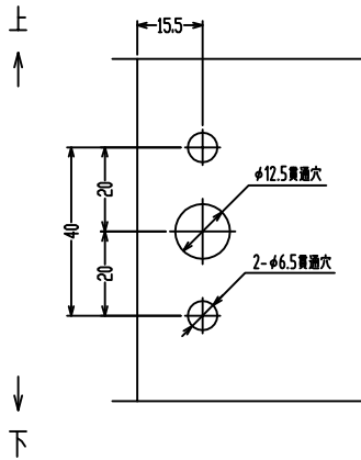
扉取付穴加工図
