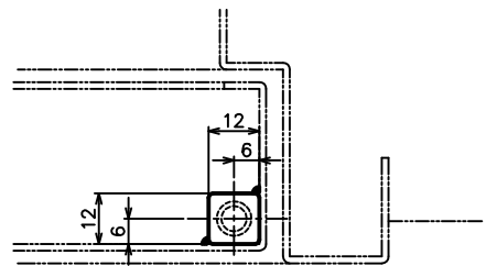
③ 下部扉ユニット
