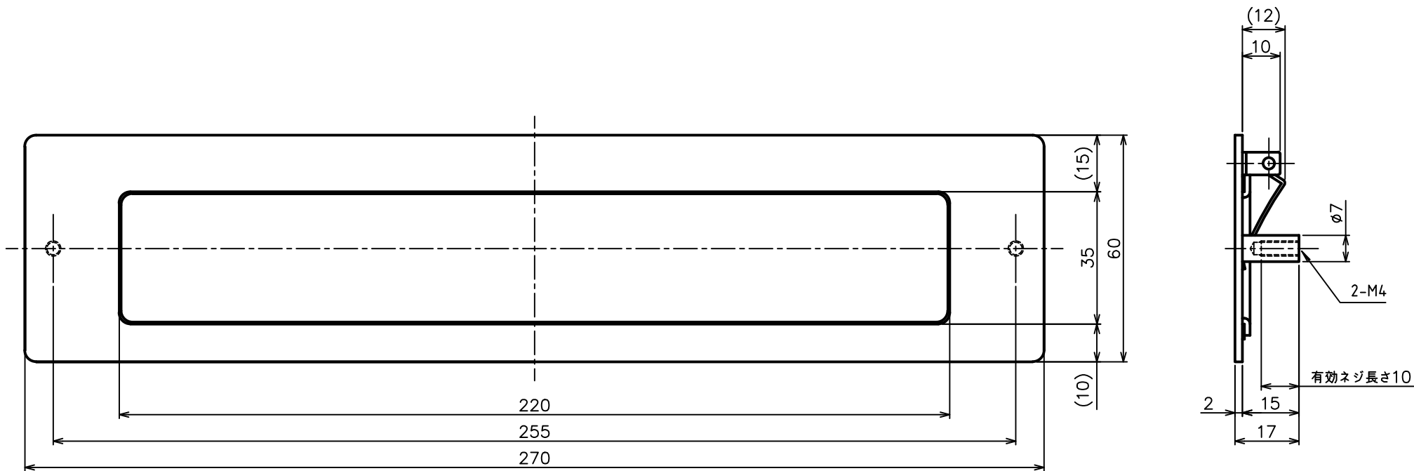
切欠き図
