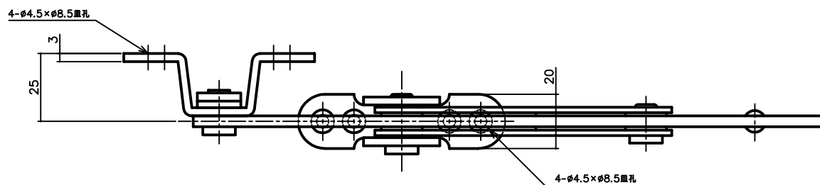
ドア90°開口時推奨取付位置
