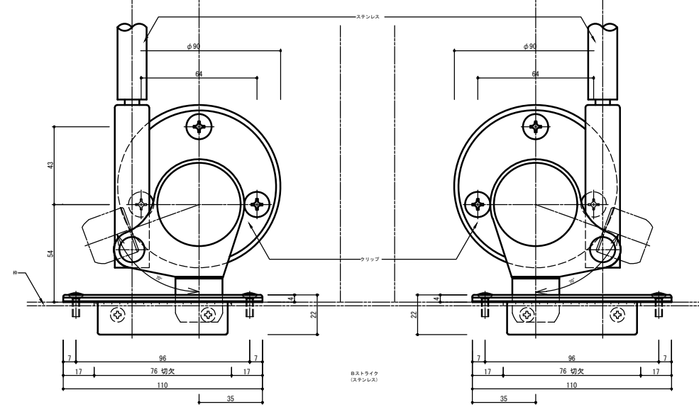
SF-2 図は右勝手(RH)を示す。
