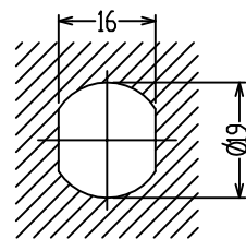
取付穴加工図
