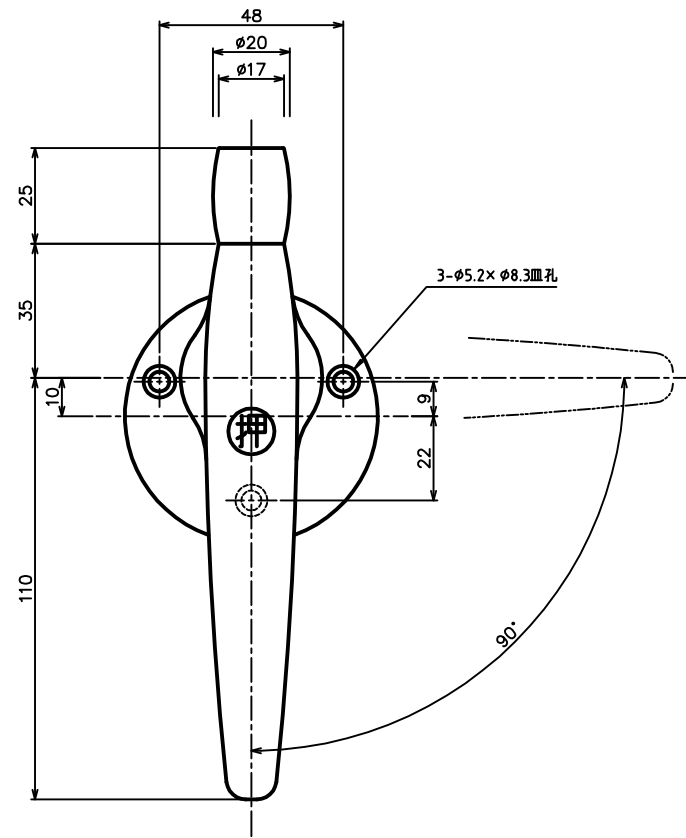
<両開き納り図>
