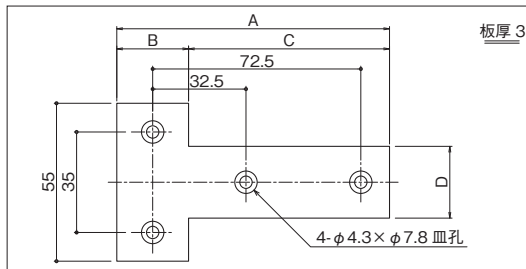
寸法表
